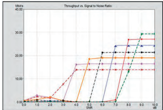
Рис. 2. Зависимость пропускной способности от отношения сигнал-шум
