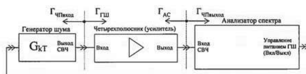
Рисунок 1б. Измерение суммарного коэффициента шума четырехполюсника в анализаторе спектра КШ чпвас
